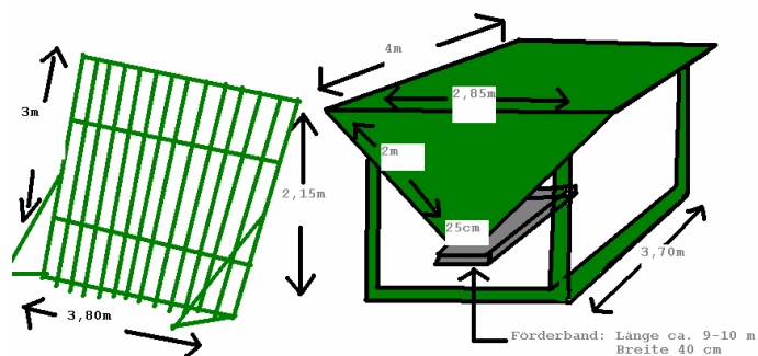
Skizze für Maße von Grünem Trichter
